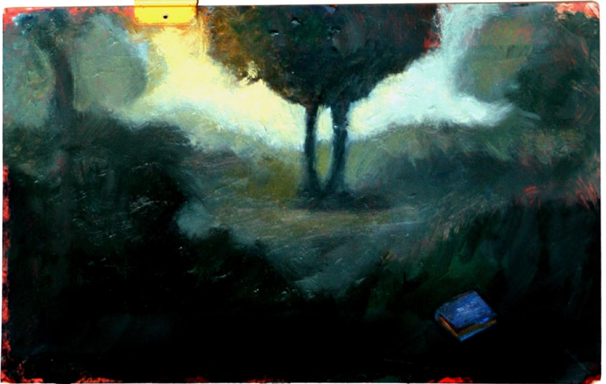
«Foucault's Pendulum»
